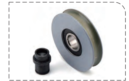
65*13*6202 Hitachi door hanger roller
