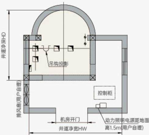
机房平面图 ROOM LAYOUT
