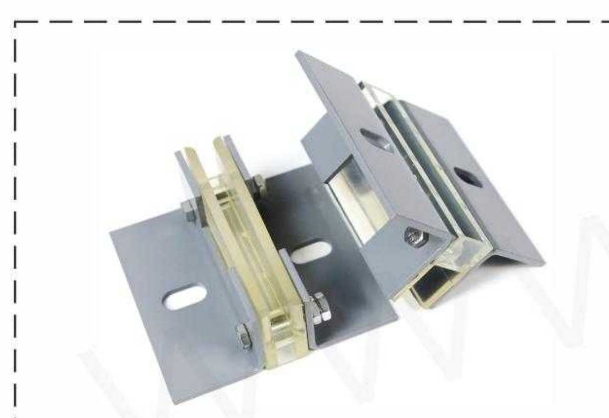
120*10/16 Otis guide shoe
