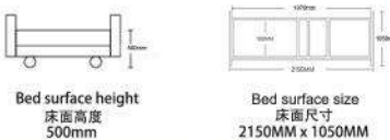
Configuration and technical parameters 配置及技术参数:
