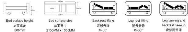
Configuration and technical parameters 配置及技术参数:
