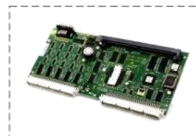
ID. NR. 591640 Schindler 5400 main board
