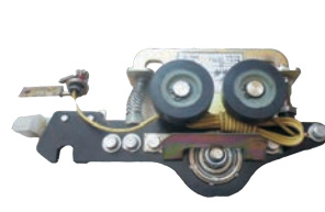
日立电梯门锁 Sp387 Hitachi elevator door lock
