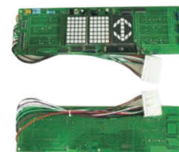
日立门眉显示板 SP001388 H ITACHI intel display board
