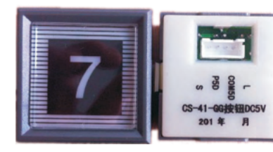
富士电梯按钮 SP167 FUJI elevator push button Sp167
