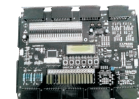
四川快速主板 Sichuan EXPRESS Main Board Int2000-s3
