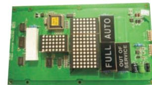
现代电梯显示板 Hyundai Display Board OPB-051 sp4090
