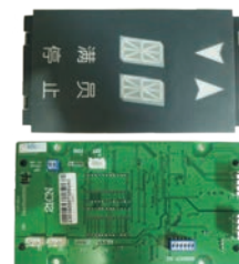
奥的斯3100显示板DAA25140NNN 14 SP001274 OTIS elevator display board 3100 DAA25140NNN14
